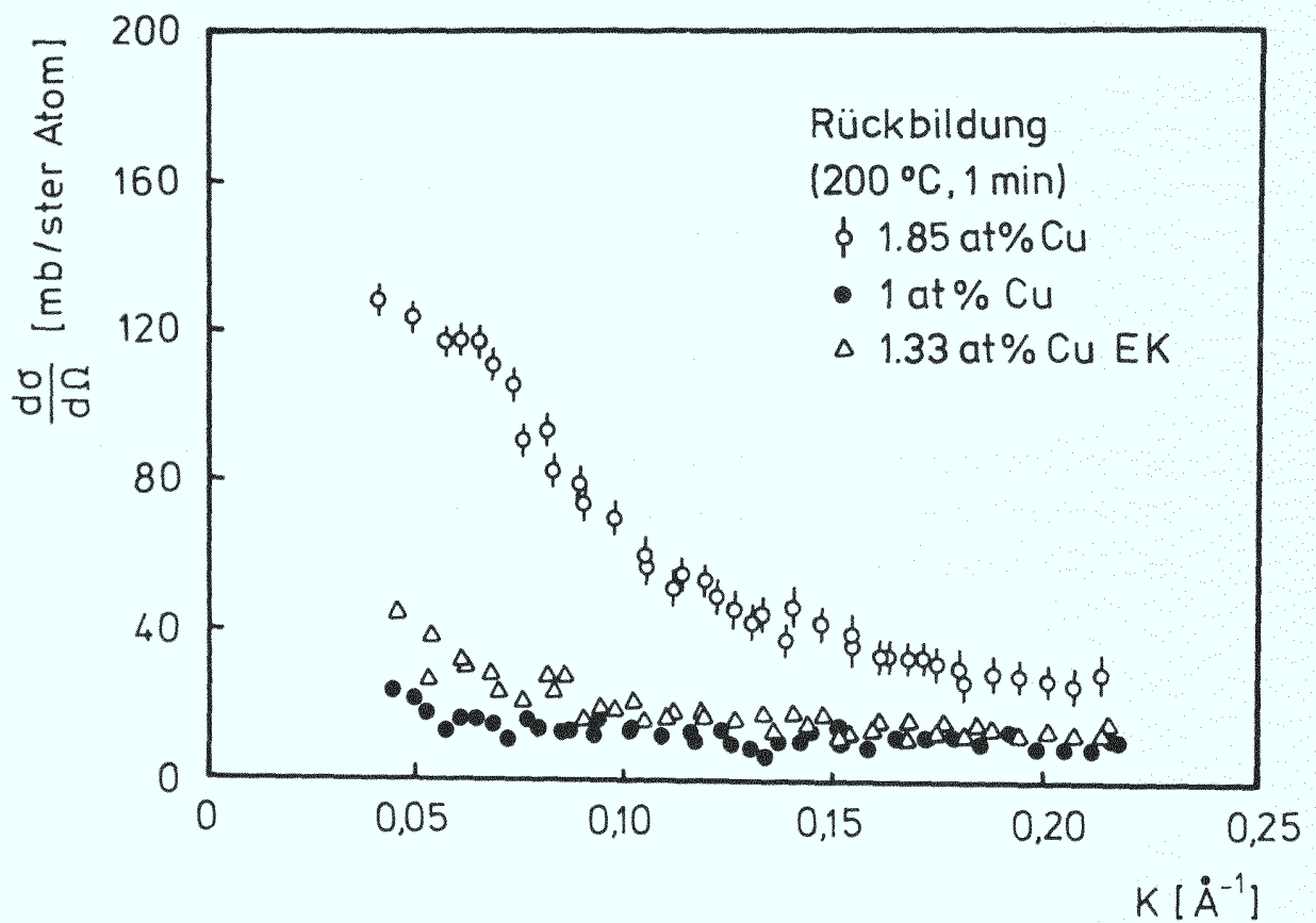
Abb. 33: Kleinwinkelstreuquerschnitt an revertierten Al Cu-Legierungen
