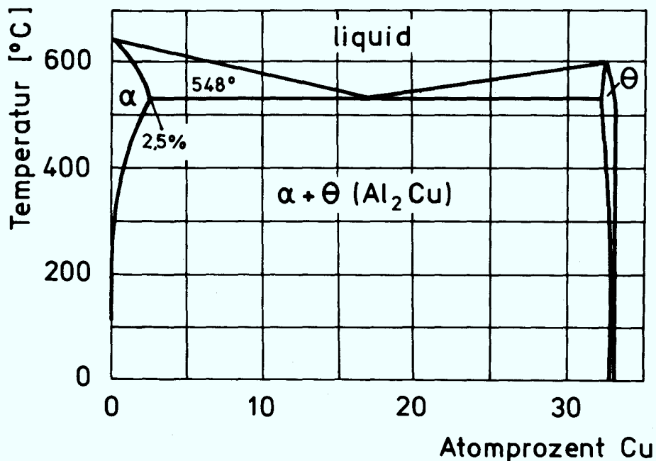
Abb. 1: Aluminiumreiche Seite des Phasendiagramms Al-Cu /2.6/
