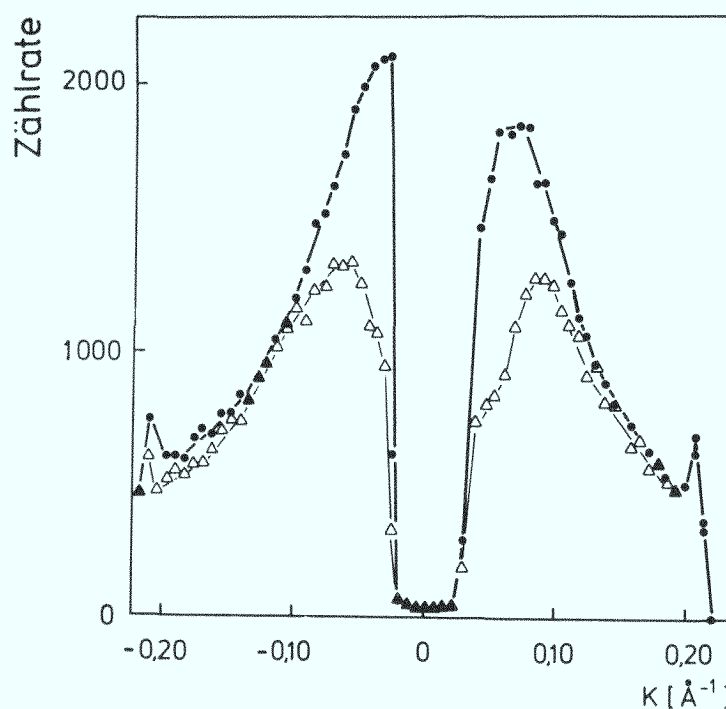
Abb. 21: Rohdaten für die KWNS an zwei AlCu-Legierungen mit 2 at% Cu, die bei Raumtemperatur (Dreiecke) bzw. bei 100 °C (Punkte) ausgelagert wurden.
