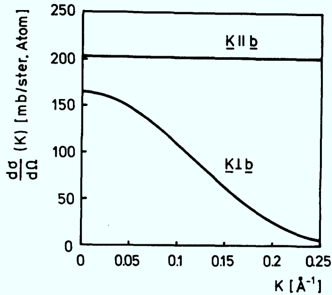
Abb. 25: Streuquerschnitt an ausgerichteten GPI-Zonen in AlCu ( X_\alpha = 1 , 2b/a\alpha = -0,30 , R = 12,5 \text{ \AA} , a = 4,0496 \text{ \AA} , v = 0,35 und c = 0,0185 )
